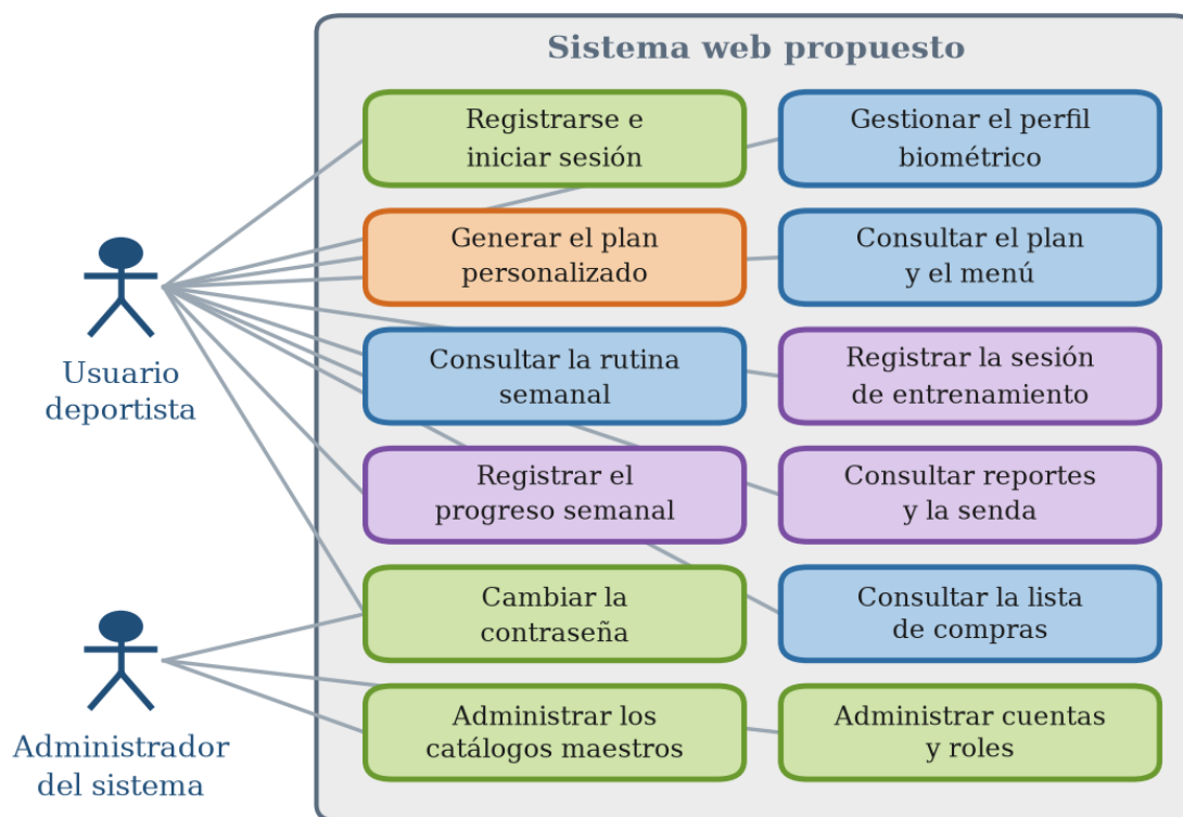
Figura 44. Diagrama de casos de uso del sistema por actor
