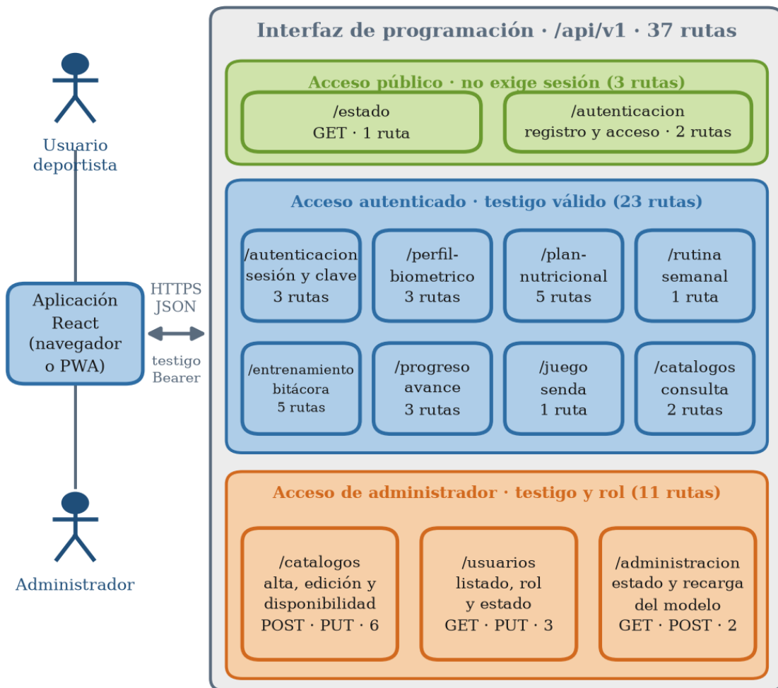
Figura 34. Diagrama de interfaces externas de la interfaz de programación de aplicaciones
