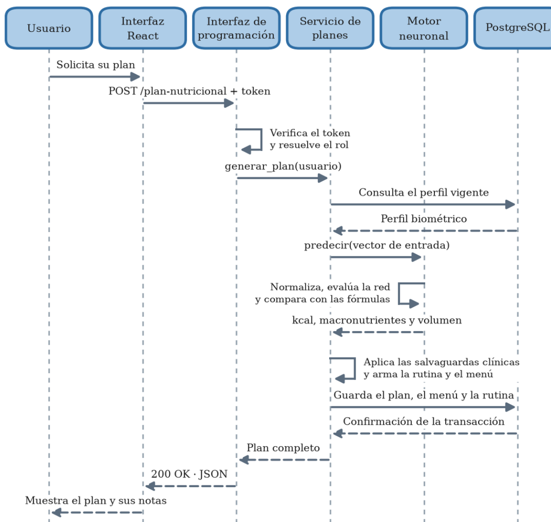
Figura 46. Diagrama de secuencia de la generación del plan nutricional
