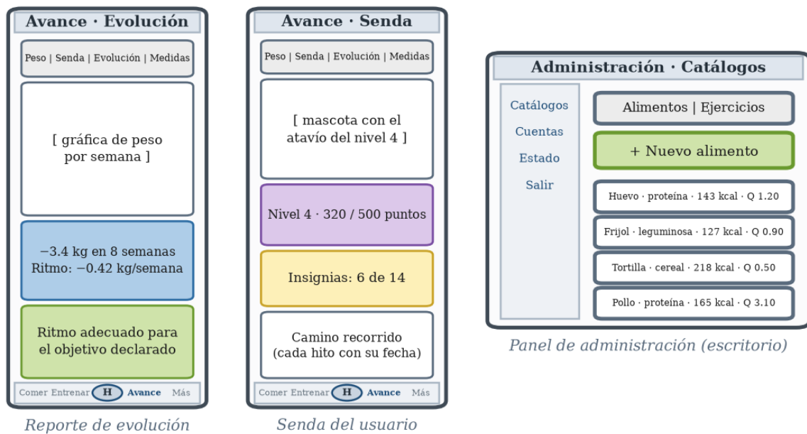
Figura 40. Prototipos de las pantallas de avance y del panel de administración
