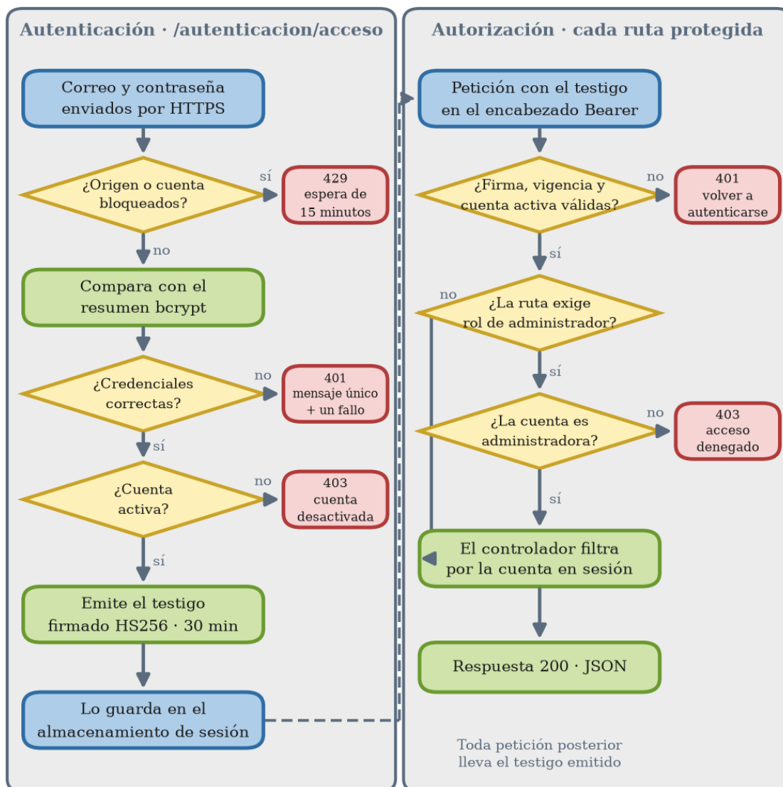
Figura 42. Diagrama de flujo de la autenticación y la autorización
