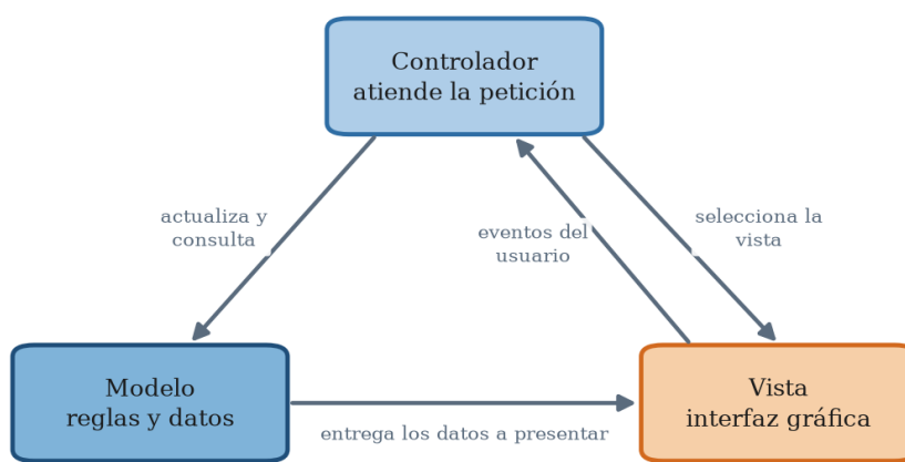
Figura 27. Patrón de arquitectura Modelo-Vista-Controlador
