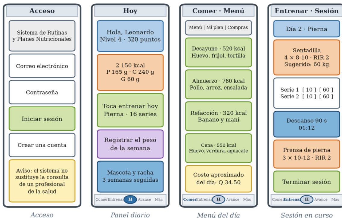
Figura 39. Prototipos de las pantallas principales del usuario deportista
