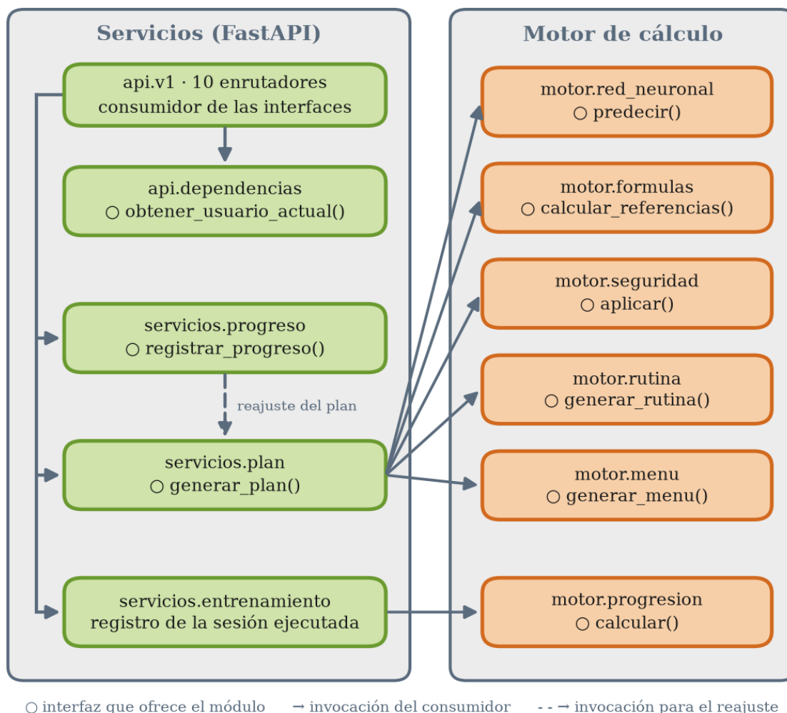
Figura 33. Diagrama de interfaces internas entre los módulos del servidor
