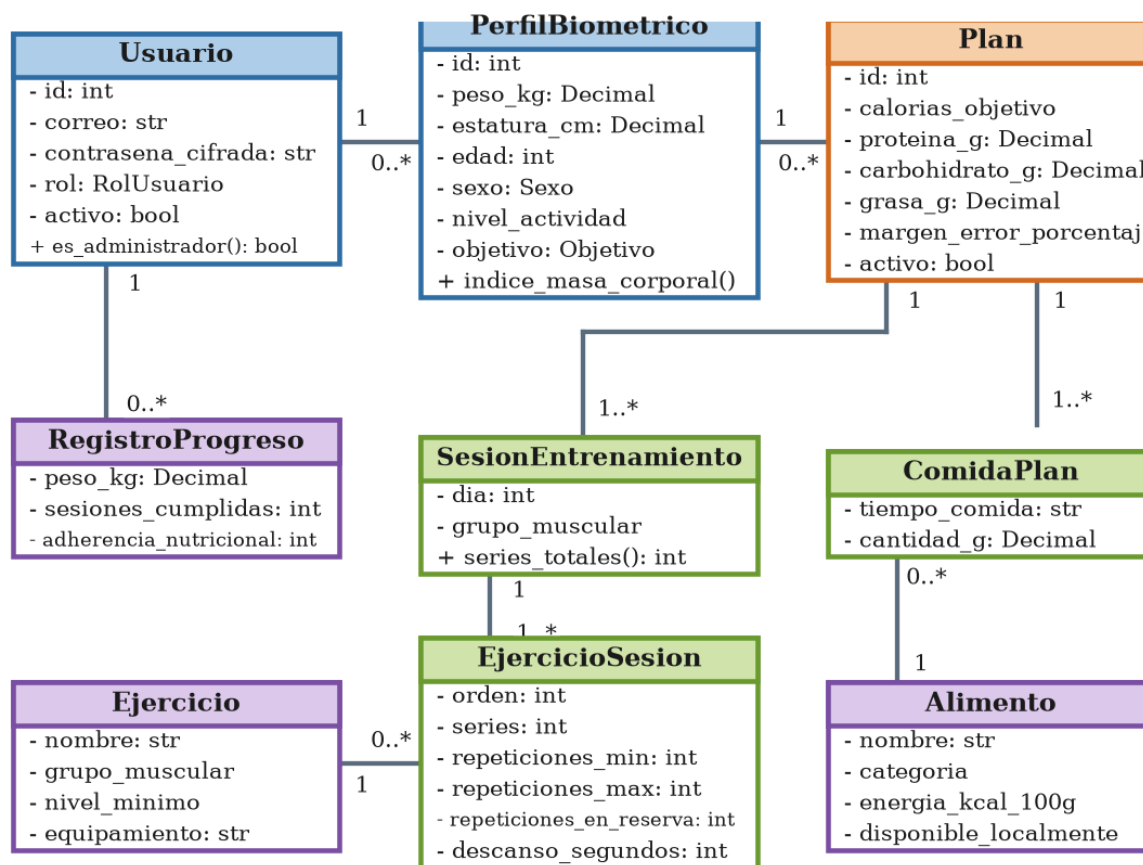
Figura 35. Diagrama de clases del dominio del sistema
