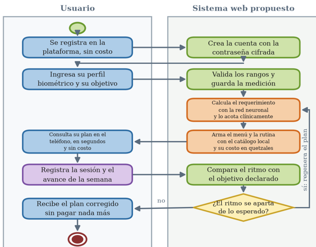
Figura 49. Proceso sistematizado para obtener un plan de nutrición y entrenamiento
