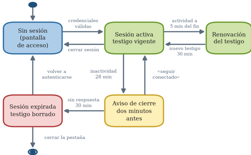
Figura 43. Diagrama de estados de la sesión del usuario
