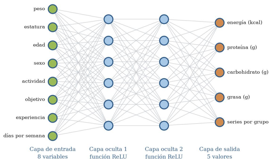
Figura 23. Estructura de una red neuronal artificial multicapa
