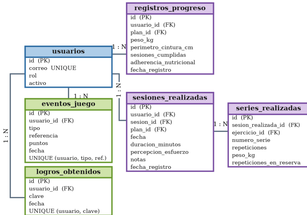
Figura 38. Modelo entidad-relación del sistema, segunda parte
